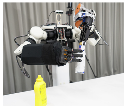
多指ハンド
