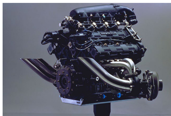
「RA166E」：FW11 に搭載された Honda 製エンジン
